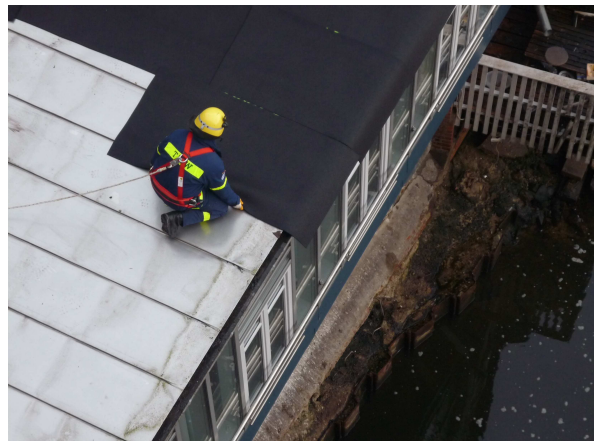
links: ein Halbponton des OV Uelzen wird einsatzbereit gemacht; rechts: Ausbringen von Schutzmatte auf dem Dach eines angrenzenden Vorbaus
